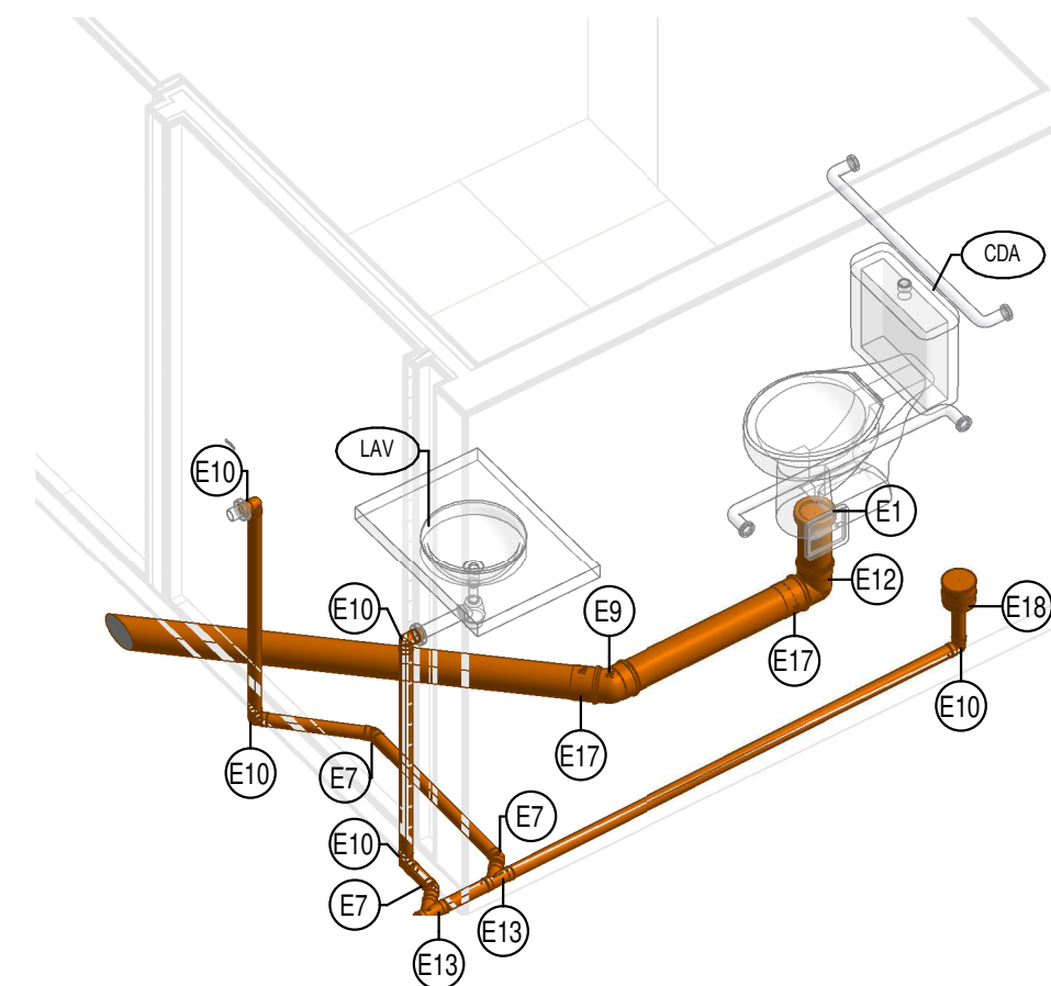
PERSPECTIVA 01 - ESGOTO
